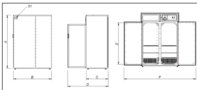
ECO3 - 1250
