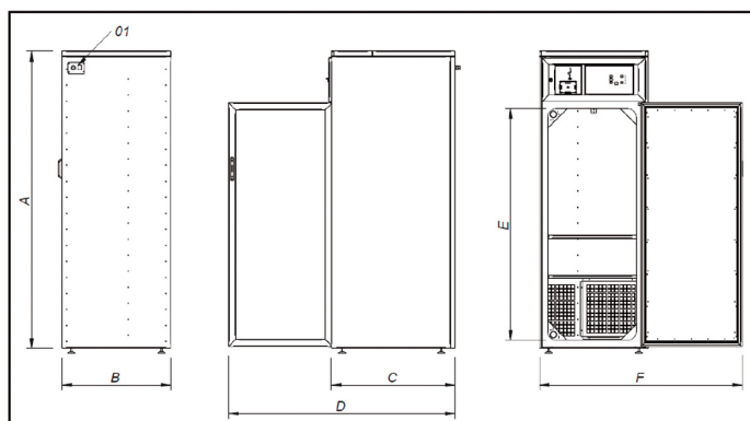
ECO3 - 300 ECO3 - 600
